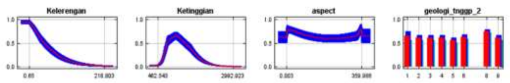
Gambar 52. Kurva respon
