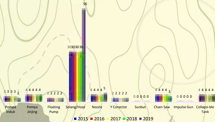
Gambar III.6. Grafik Sarana Peralatan Mekanik Pengendalian Kebakaran Hutan Tahun 2014 - 2018
