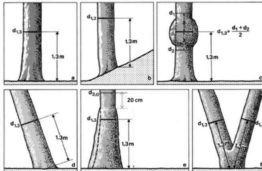
Gambar 12 Pengukuran Diameter
